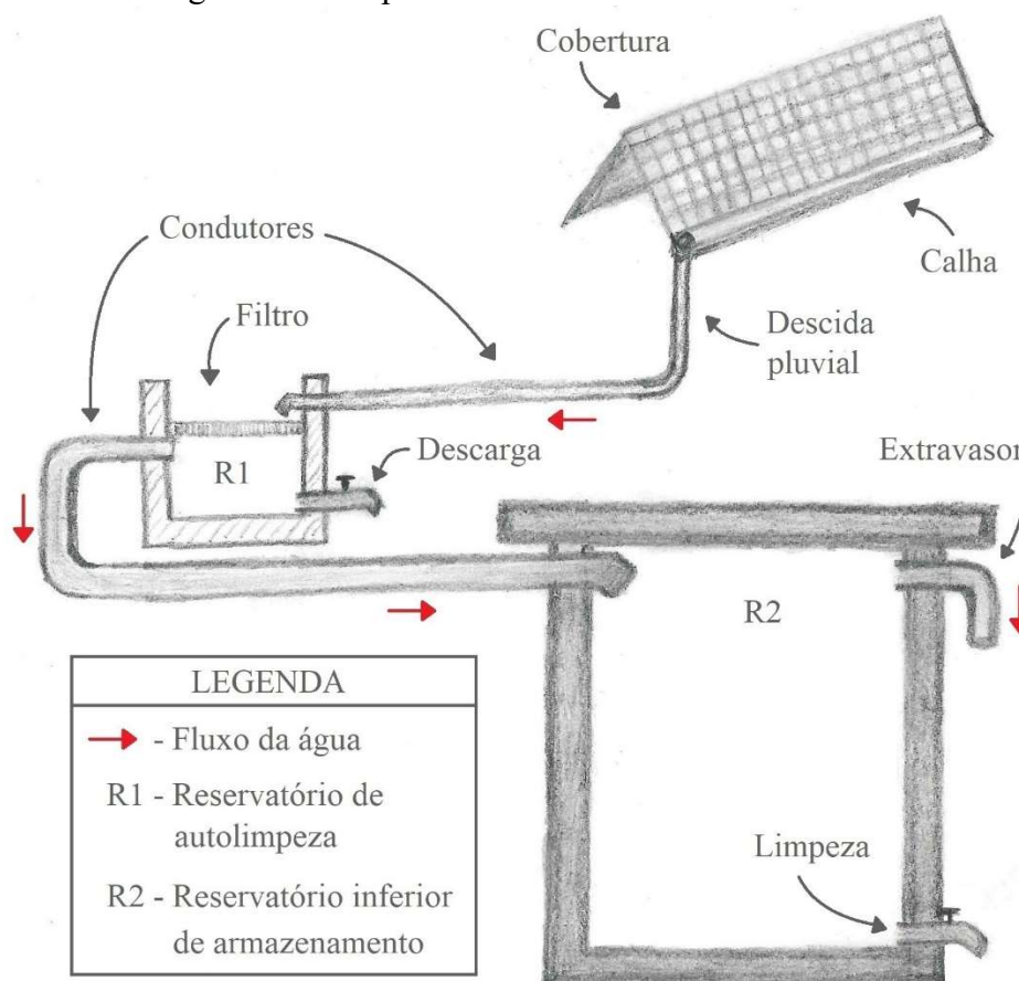
Figura 1 – Componentes de um sistema convencional
