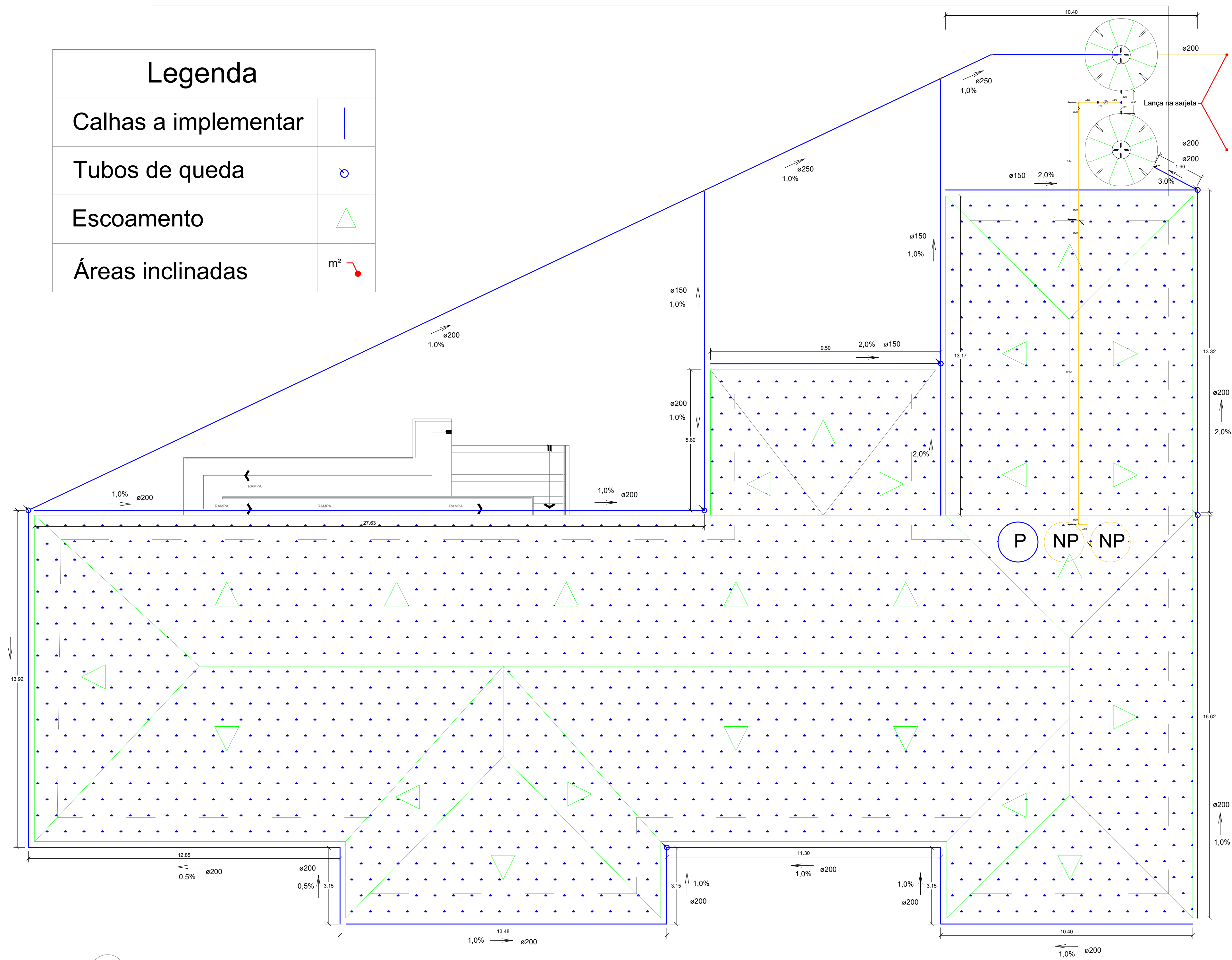
03 Planta de Cobertura: Cenário 02 e 03 - Esc.: 1/100
