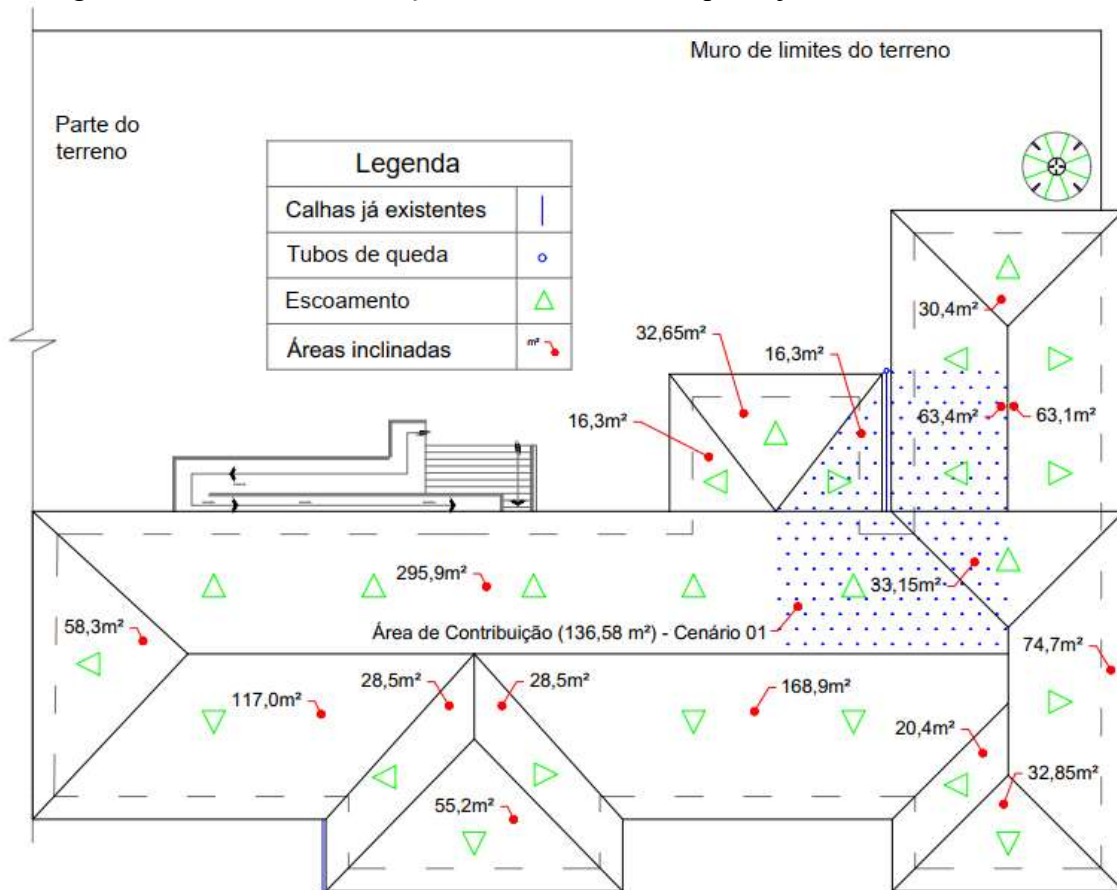
Figura 9 – Área de contribuição, calhas e tubos de queda já existentes – Cenário 01
