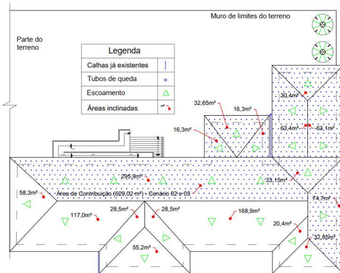
Figura 10 – Área de contribuição, calhas e tubos de queda – Cenários 02 e 03
