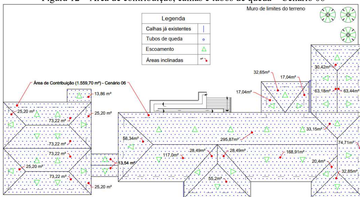
Figura 12 – Área de contribuição, calhas e tubos de queda – Cenário 06
