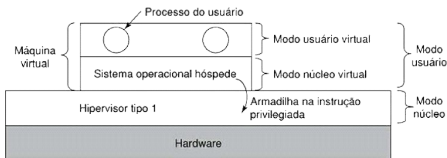
Figura 2 – Hipervisor tipo 1
