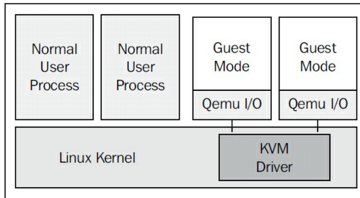
Figura 4 – Interação entre o QEMU e o KVM
