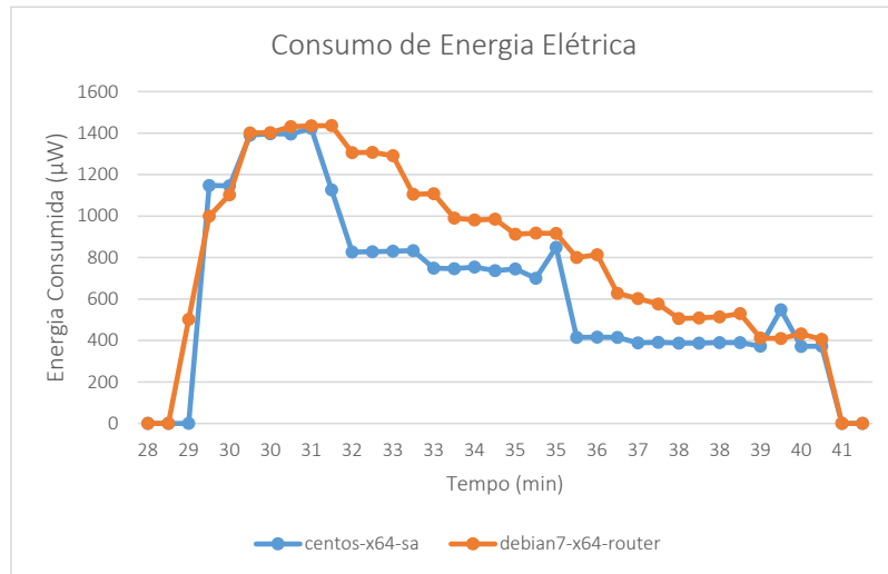
Figura 10 – Gráfico dos consumos energéticos das máquinas virtuais centos7-x64-sa e debian-x64-router
